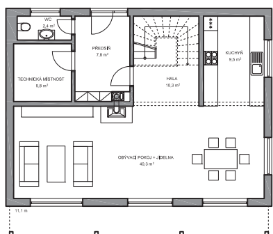
Přízemí
